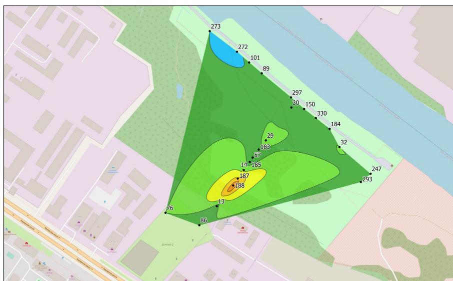
Рис. 2.4.9 Схема горизонтальных смещений приповерхностной зоны грунтов на участке Коломенское за период 2017-2022 гг.
