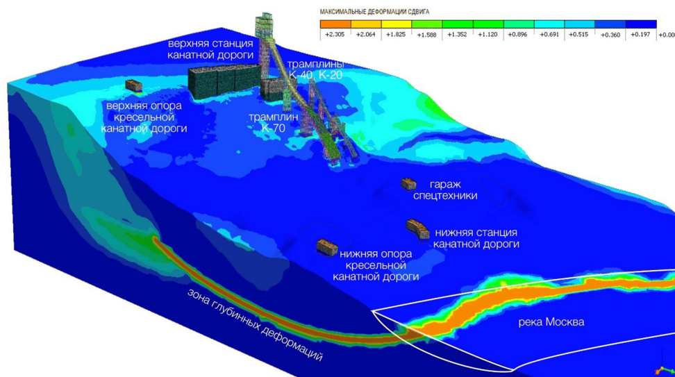
Рис. 24.8 Зоны формирования потенциальных сдвиговых деформаций
