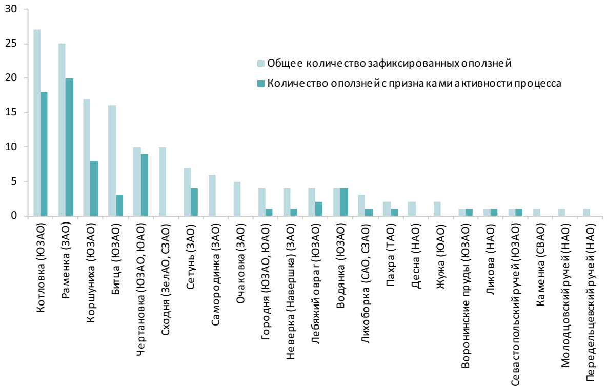
Рис. 2.4.17 Распределение активных форм оползней в долинах малых рек
