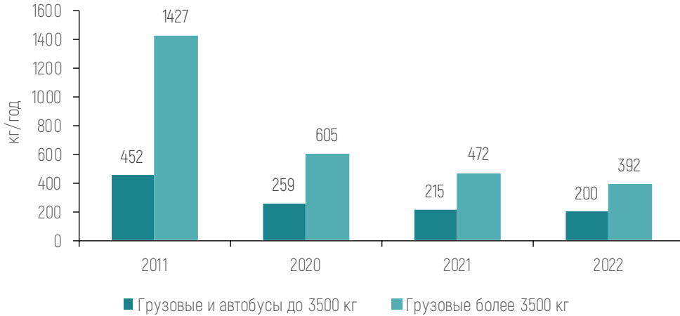
Рис. 4.113 Изменение средних годовых выбросов среднестатистического грузового автомобиля в городе Москве (Экспертная оценка, основанная на методике Распоряжения Росприроднадзора от 13.12.2019 № 37-р на основе данных ОАО «Автомобильная статистика» о распределении транспорта по экологическим классам)
