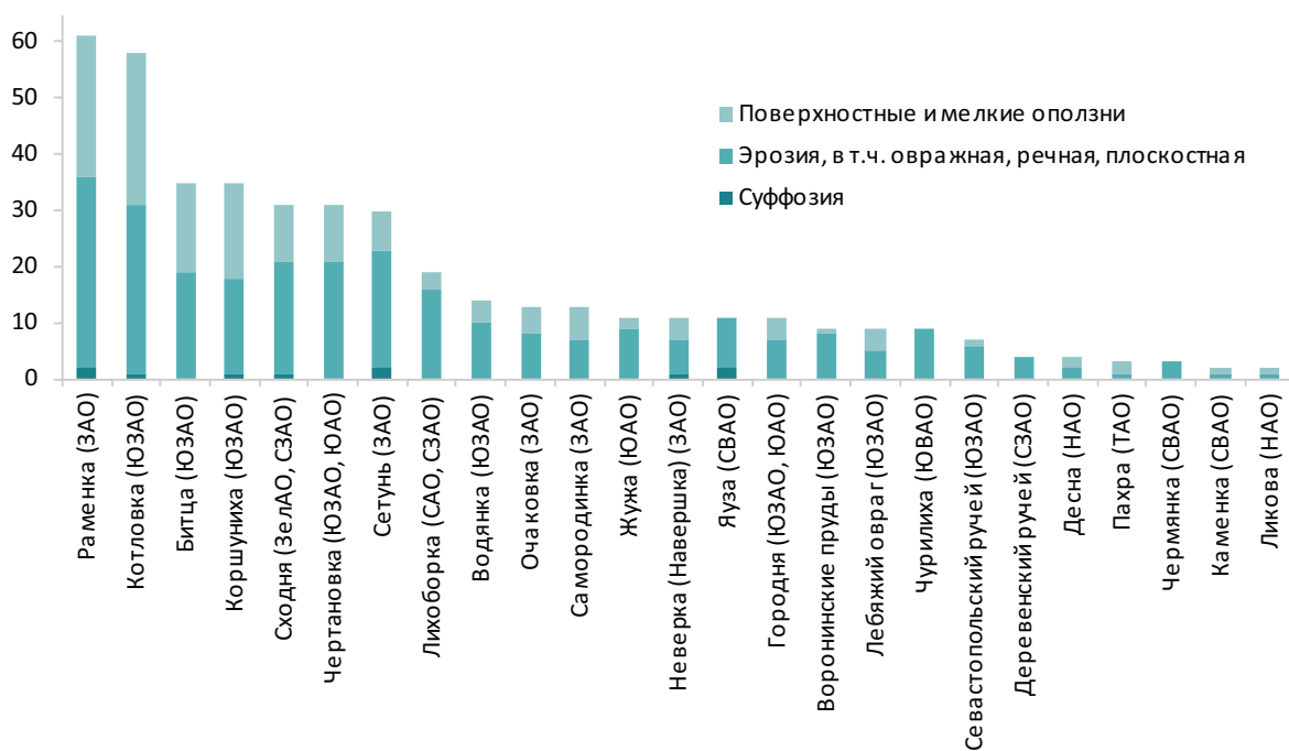
Рис. 2.4.15 Распределение типов опасных геологических процессов в долинах малых рек
