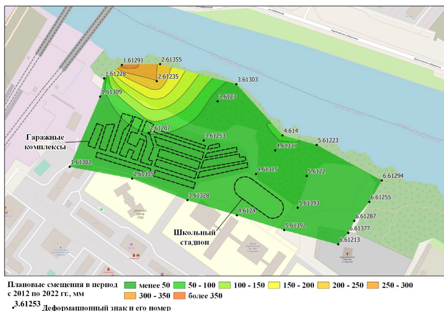
Рис. 2.4.12 Схема горизонтальных смещений приповерхностной зоны грунтов на оползневом участке Москворечье за период 2012-2022 гг.
