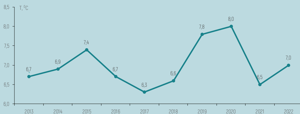
Рис. 5.1.3 Изменение средней годовой температуры воздуха в Москве за период с 2013 по 2022 гг.
