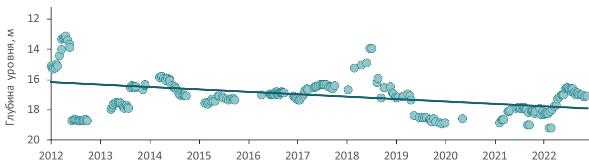
Рис. 2.5.2 Характерный график многолетних изменений уровня грунтовых вод
