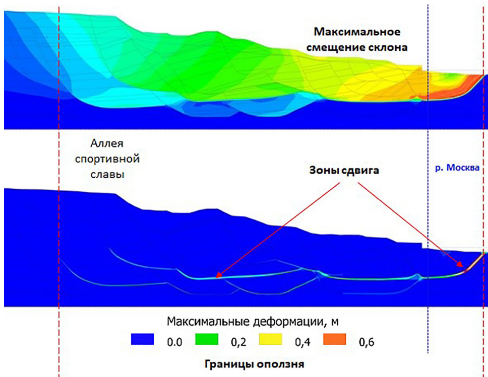
Рис. 24.7 Распределение деформаций массива грунтов по результатам моделирования
